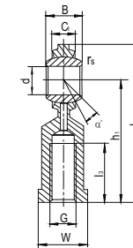
Type SIZJ ...
