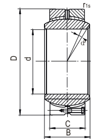
Type GEH...HC
