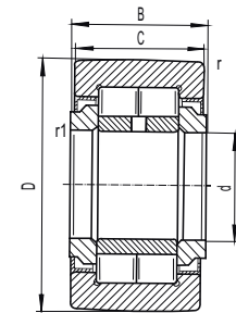
Type NUTR
