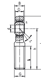
Type SAJK...C
