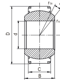
Type GEH...XT-2RS
