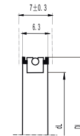
Type DX400Z2
